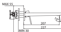
MONTECARLO Bateria umywalkowa podtynkowa ścienna
